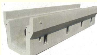
プレキャスト雨水浸透側溝
