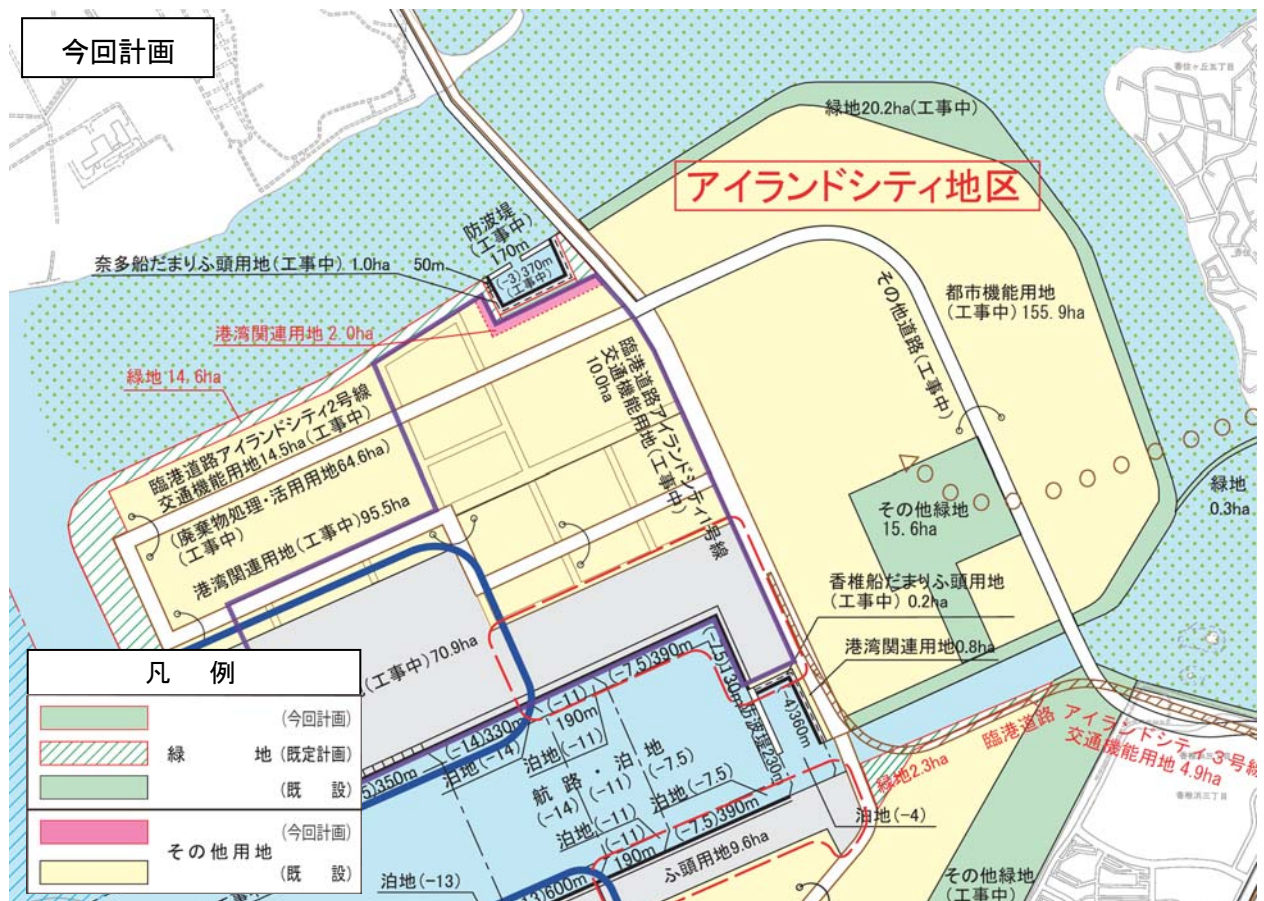
図 2 - 2 港湾計画図 (今回計画)
