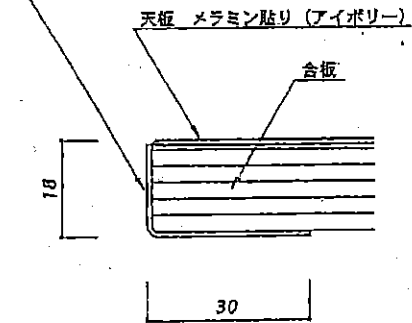
天板断面図
