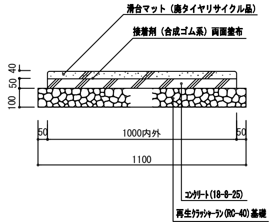
断面図 1/20
