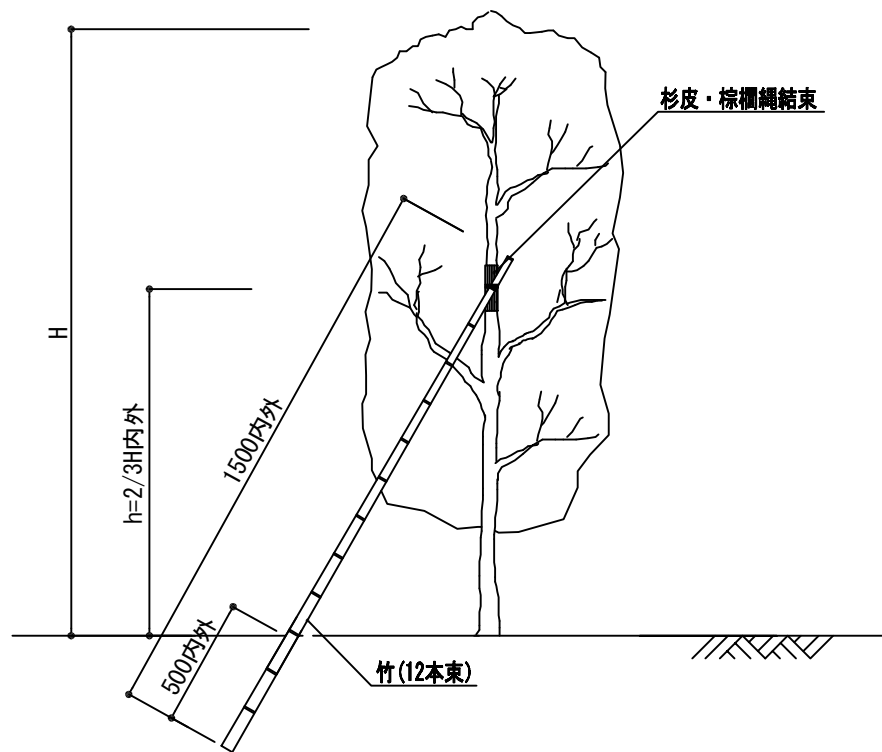
立面図
