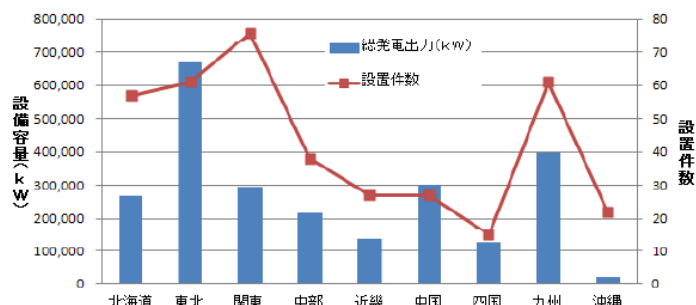
図 2-52 RPS法認定の風力発電施設のブロック別構成 出典)クール九州プロジェクト STAGE2010(経産省,九州経済産業局)
