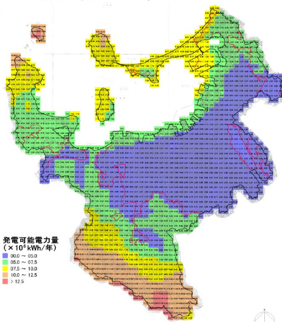
図 2-51 福岡市の小型風車設置による発電量 出典)「緑の分権改革」推進事業委託業務報告書(福岡市)
