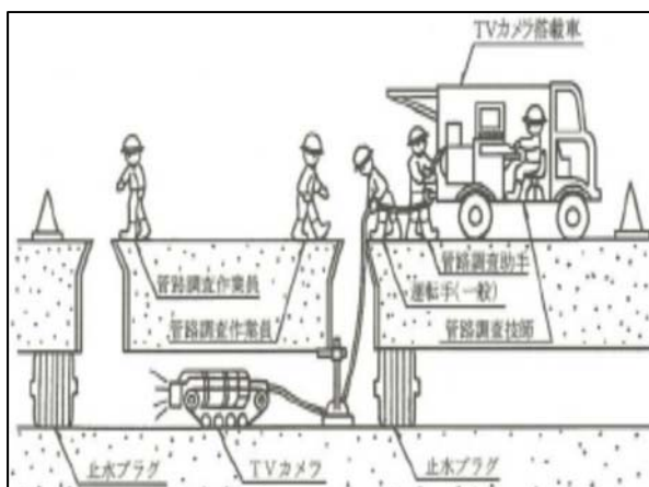
TVカメラによる管内調査 ( (公社) 日本下水道管路管理業協会 )
