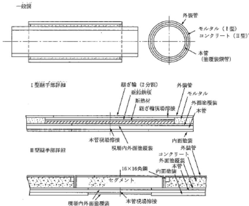
図 6-21 水道用推進鋼管
