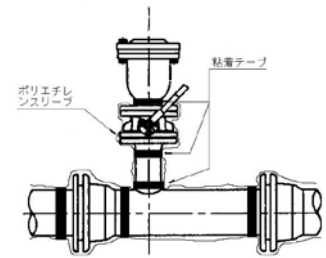
(空気弁)
