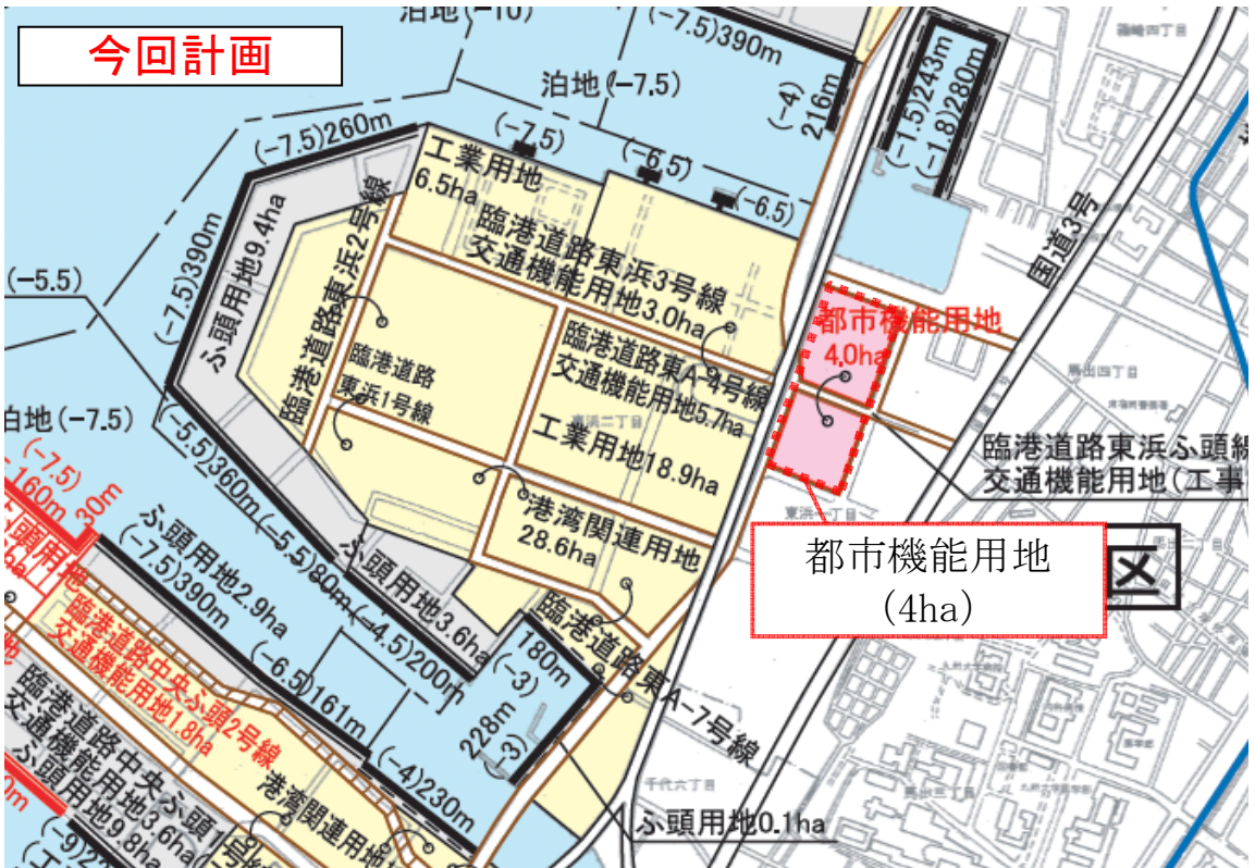
図1-2 港湾計画図の変更について（東浜ふ頭地区）
