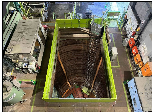
① 発進立坑の内部（深さ 21.5m）
