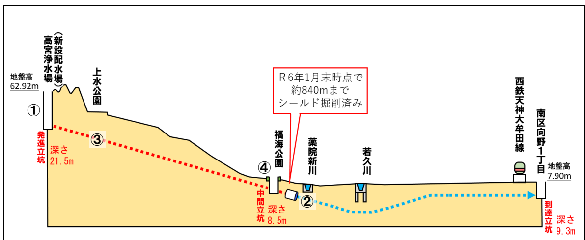
工事縦断面図
