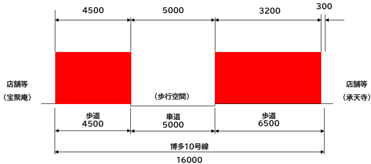
<標準断面図(歩道活用時)>
