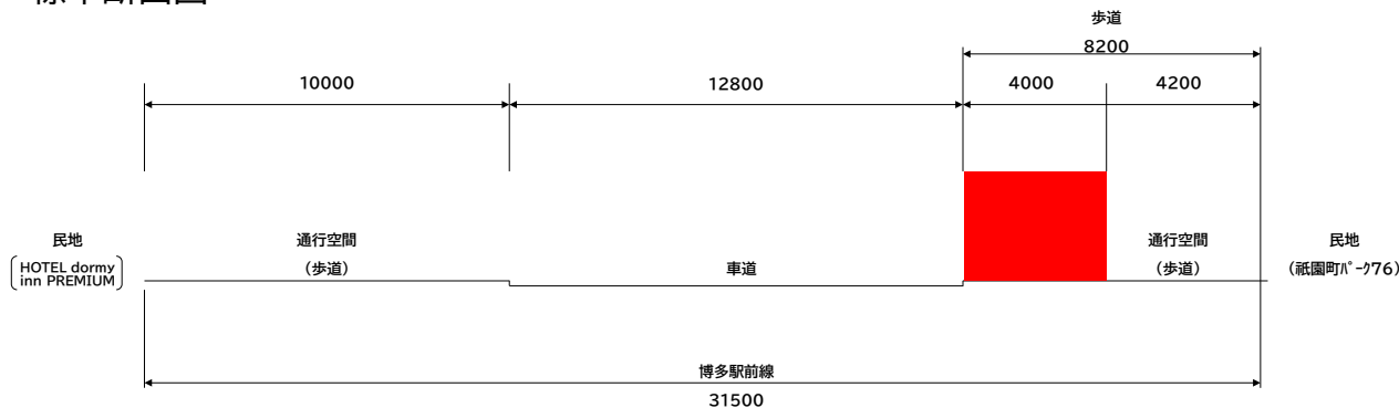
<標準断面図>
