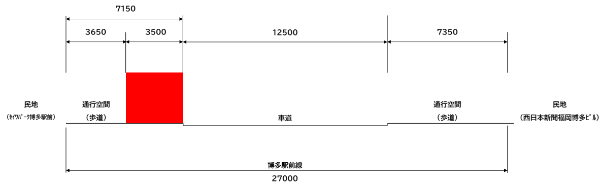
<標準断面図>
