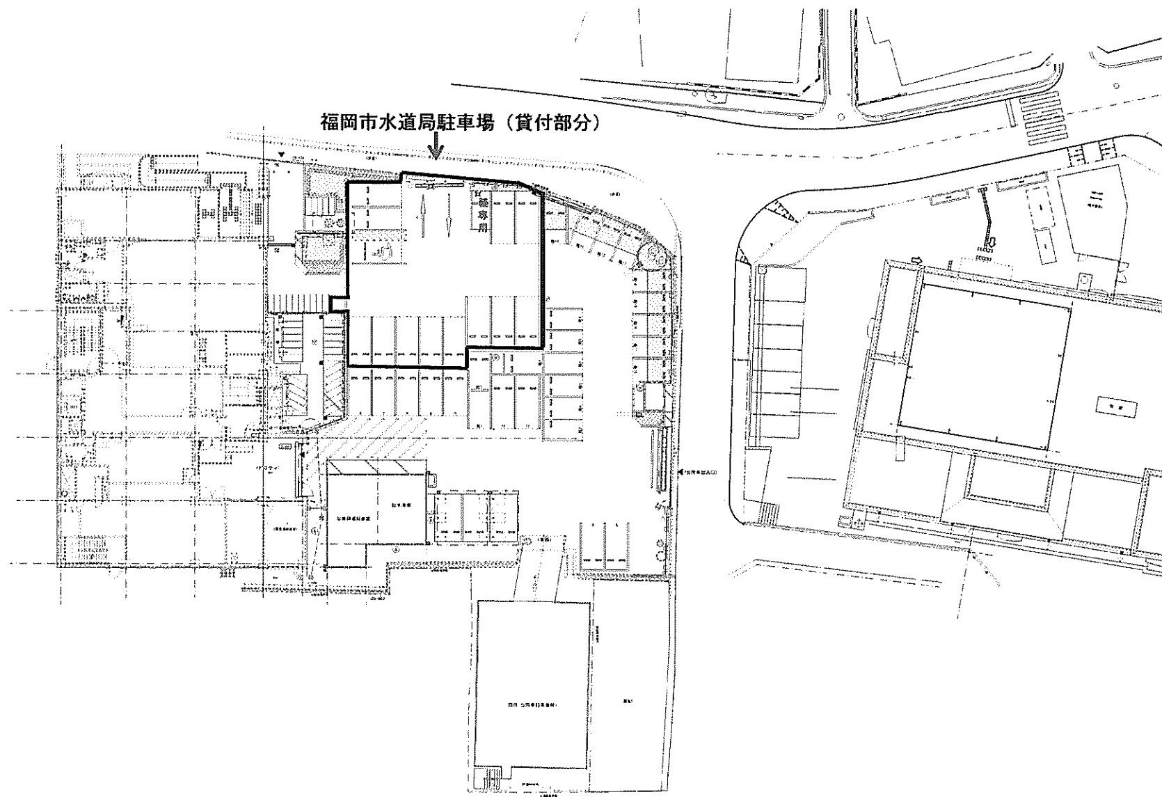
【 駐車場 図面 】
