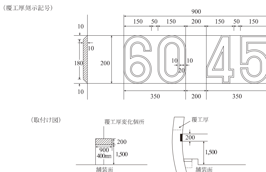
図10-6-1 覆工厚変化箇所の刻示標準図
