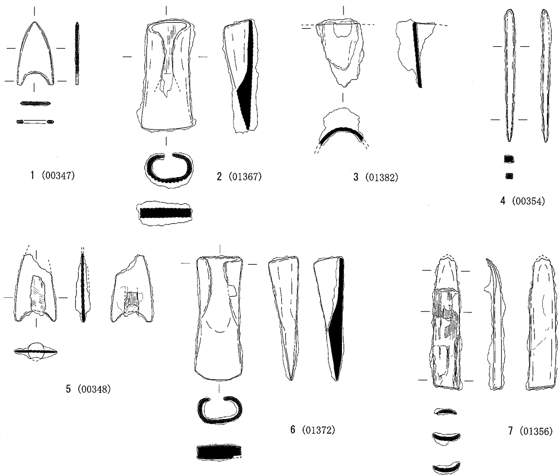
第2図 SC-060 (1~3)・074 (4~7) 出土鉄器実測図 (S=1/2)
