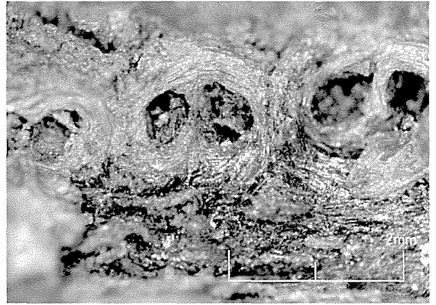
4. 羽根戸N21号墳出土鉄刀柄巻の顕微鏡写真
