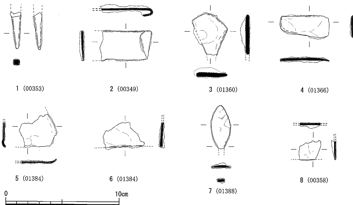
第3図 その他の遺構出土鉄器実測図 (S=1/2)
