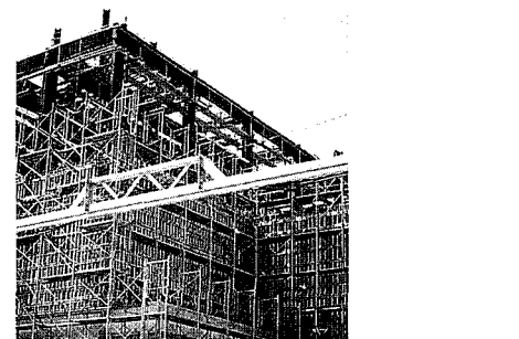
10. 二階型枠建て込み状況（平成10年3月31日）
