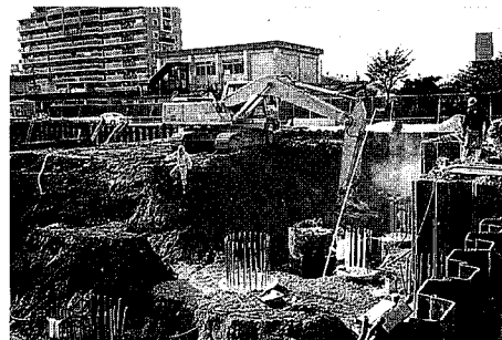
4. 根切り・床付け状況（平成9年9月30日）
