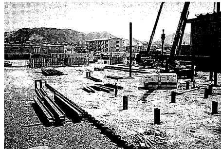
3. 土留施工状況（平成9年8月31日）
