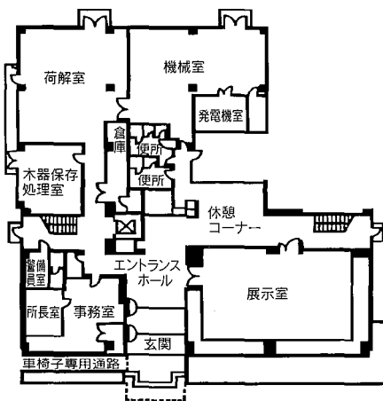
1階平面図
