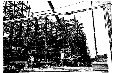
8. 鉄骨建方状況（平成10年1月31日）
