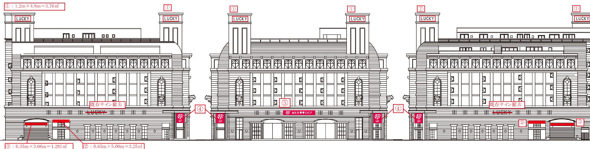
西側立面図
