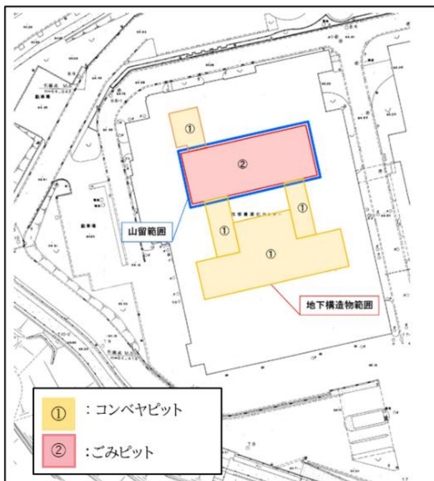
図 5.4.1 1FL 下部解体撤去構造物
