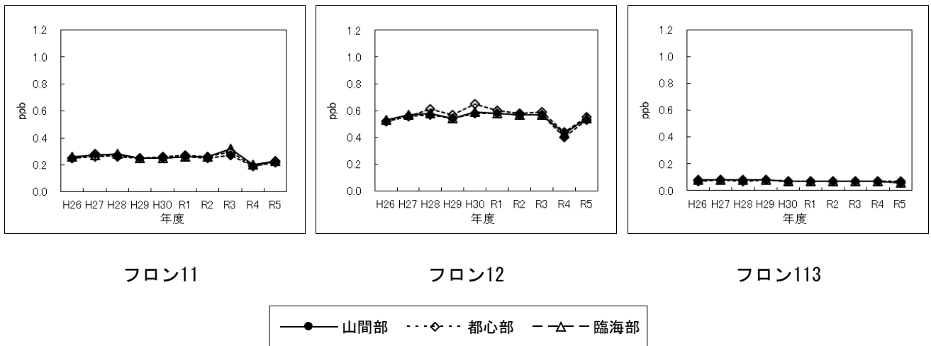
フロン濃度の推移
