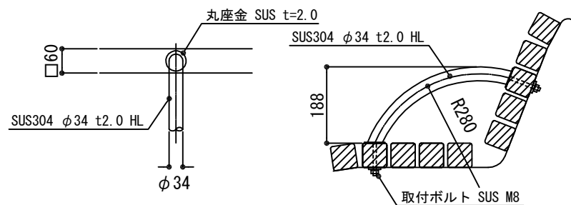
手摺取付詳細図
