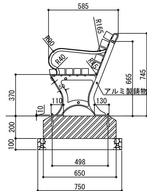
側面図
