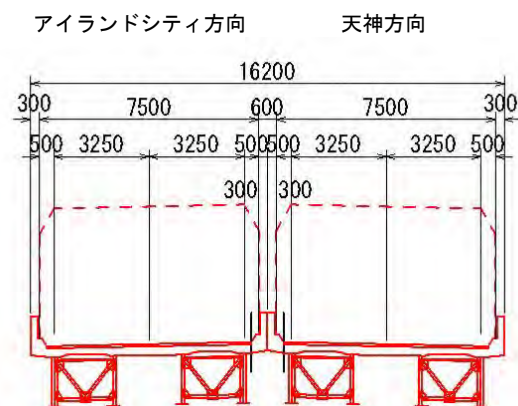
図 1-3-4 標準断面図
