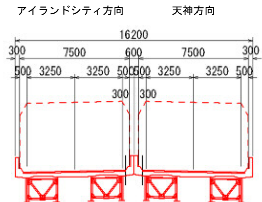
図 1-3-4 標準断面図
