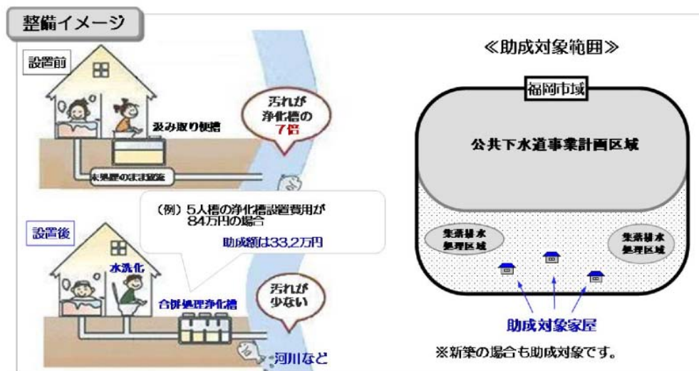
図 2.5.6 合併処理浄化槽設置助成制度による水洗化の促進
