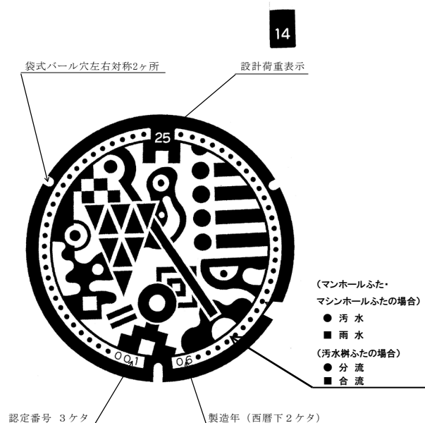
蓋表面図
