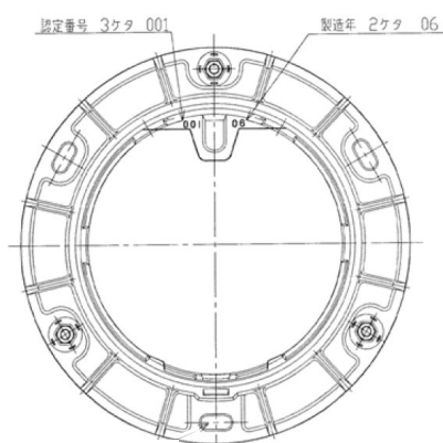
マシンホール・汚水枡ふた受枠
