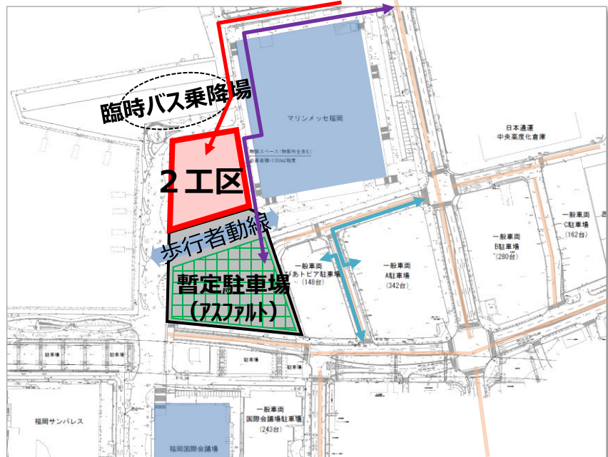
② 2工区施工時（H30.12頃）
