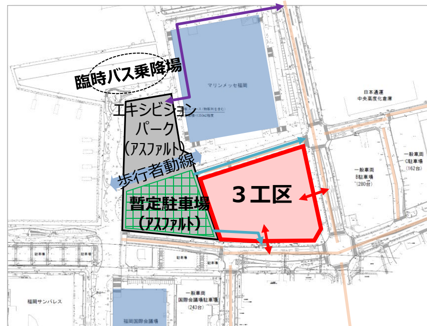
③ 3工区施工時（H31.1頃～H31.6頃）
