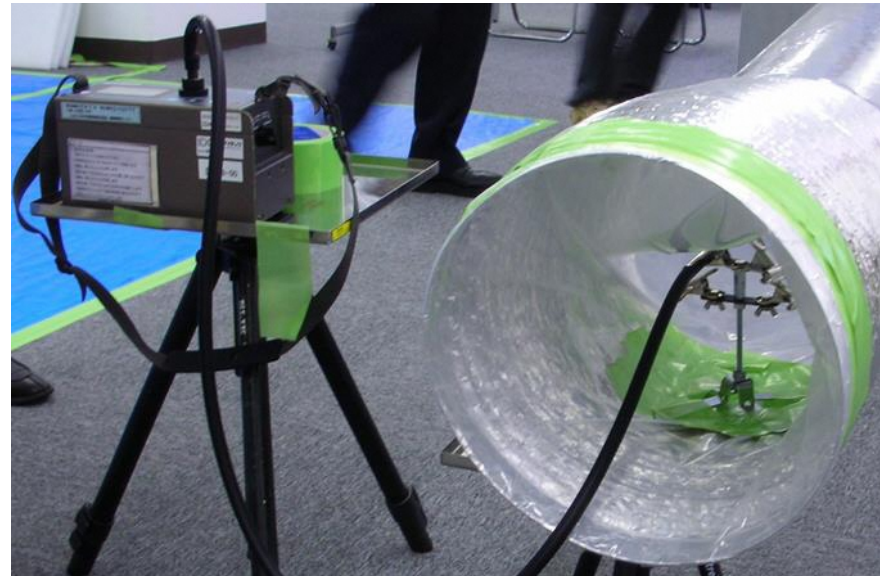
②集じん・排気装置が正常に稼働していることの確認方法の例(粉じん計による確認)
