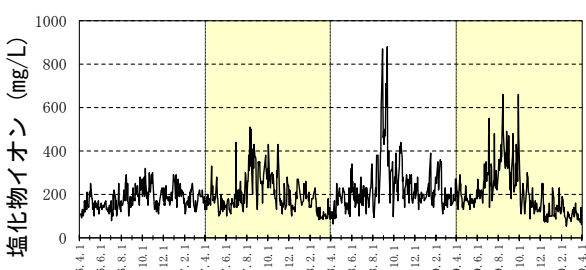
注) 図中の 塩化物イオンは流入水の日常試験結果である。
