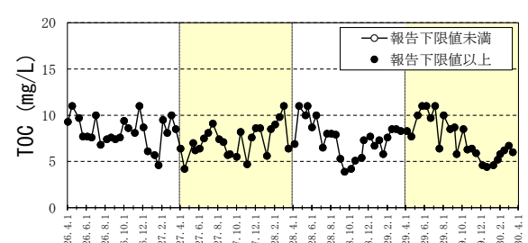
注) 図中の TOC は終沈流出水の精密試験結果である。
