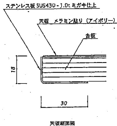
天板断面図
