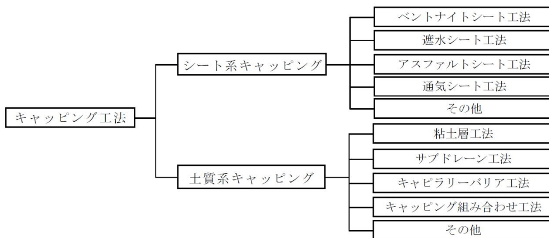
図 3.7.3 キャッピング工法の分類
