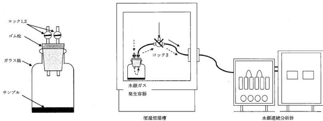
図2-2 a) 水銀ガス発生容器
