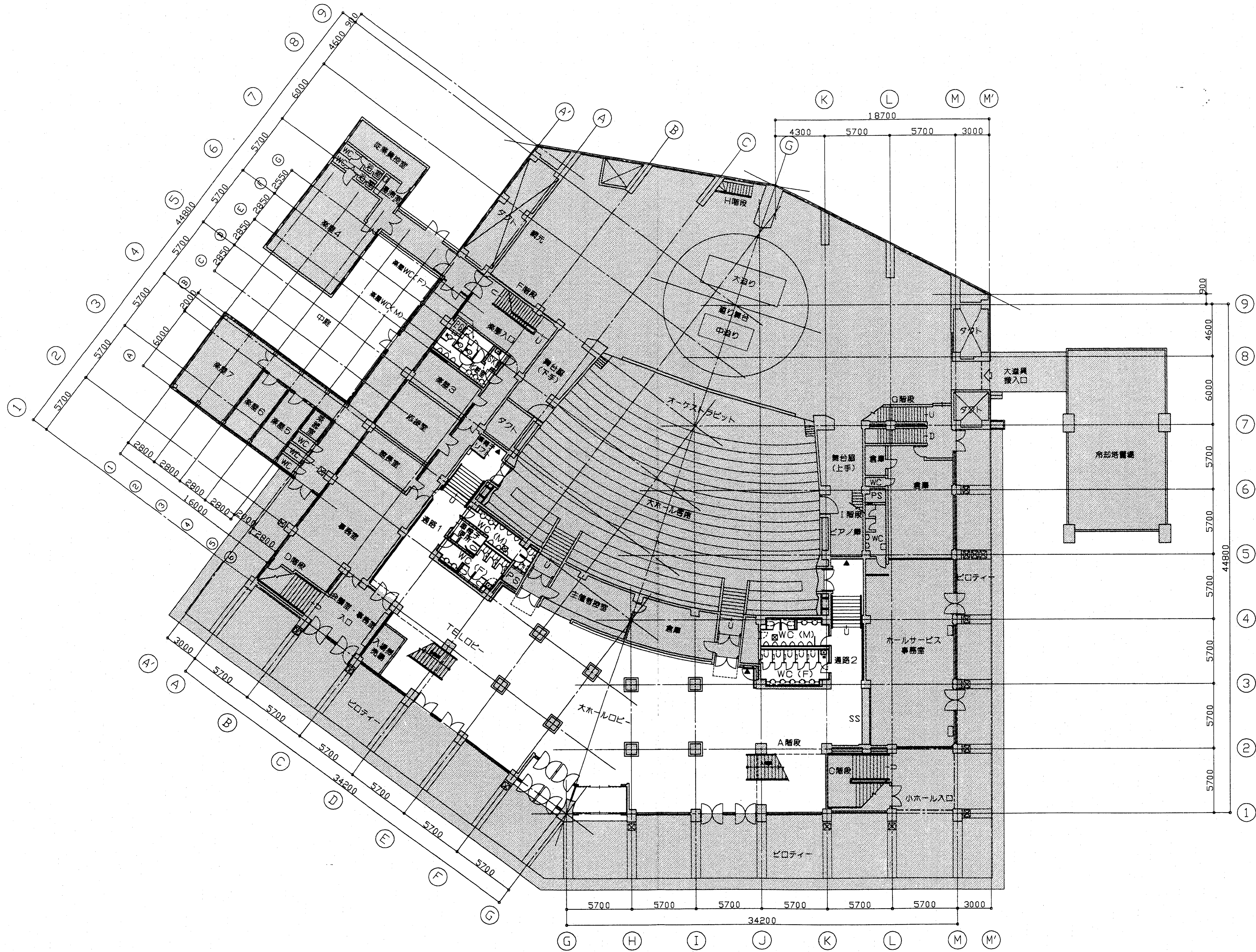
1階平面図
