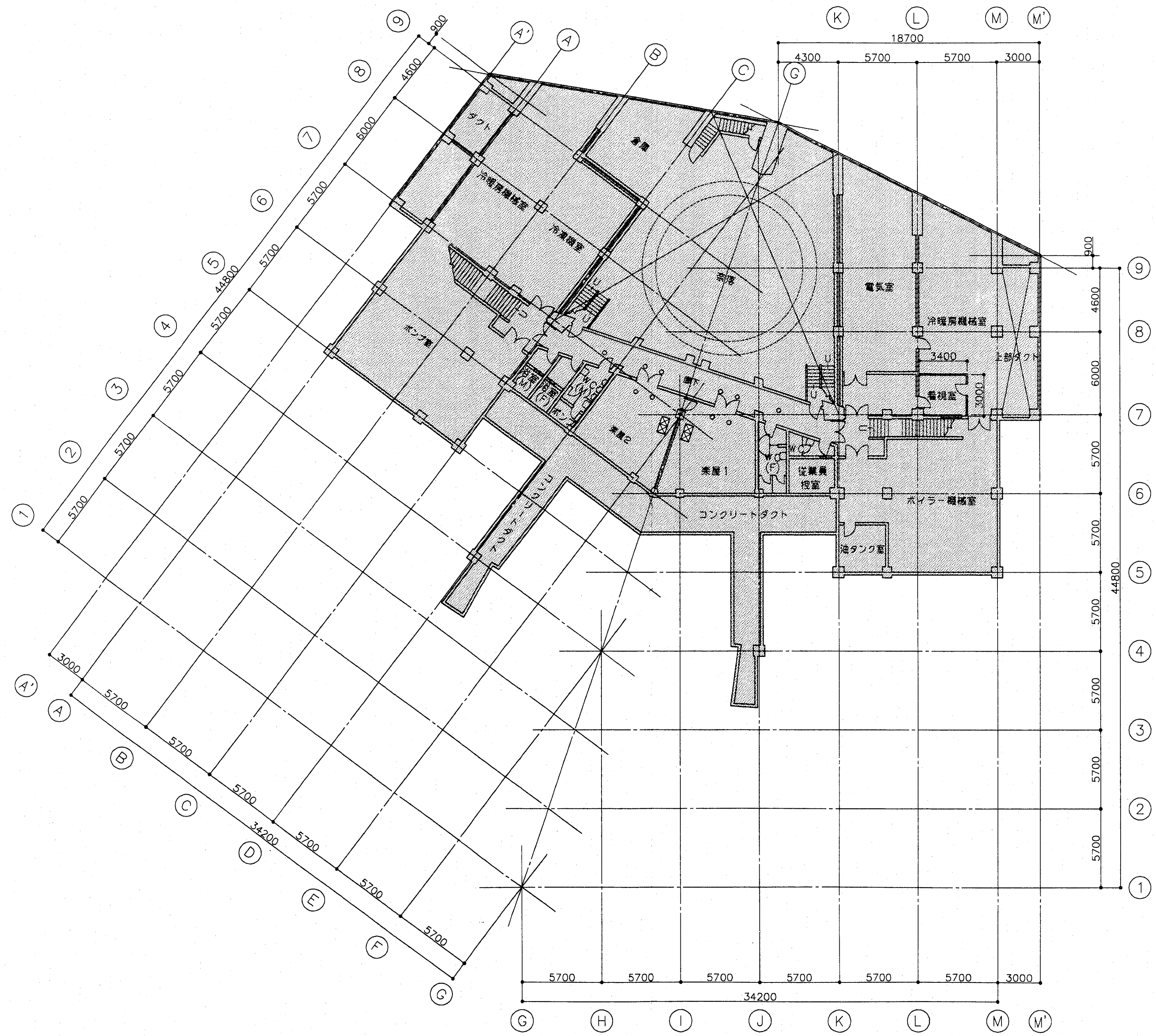
地階平面図
