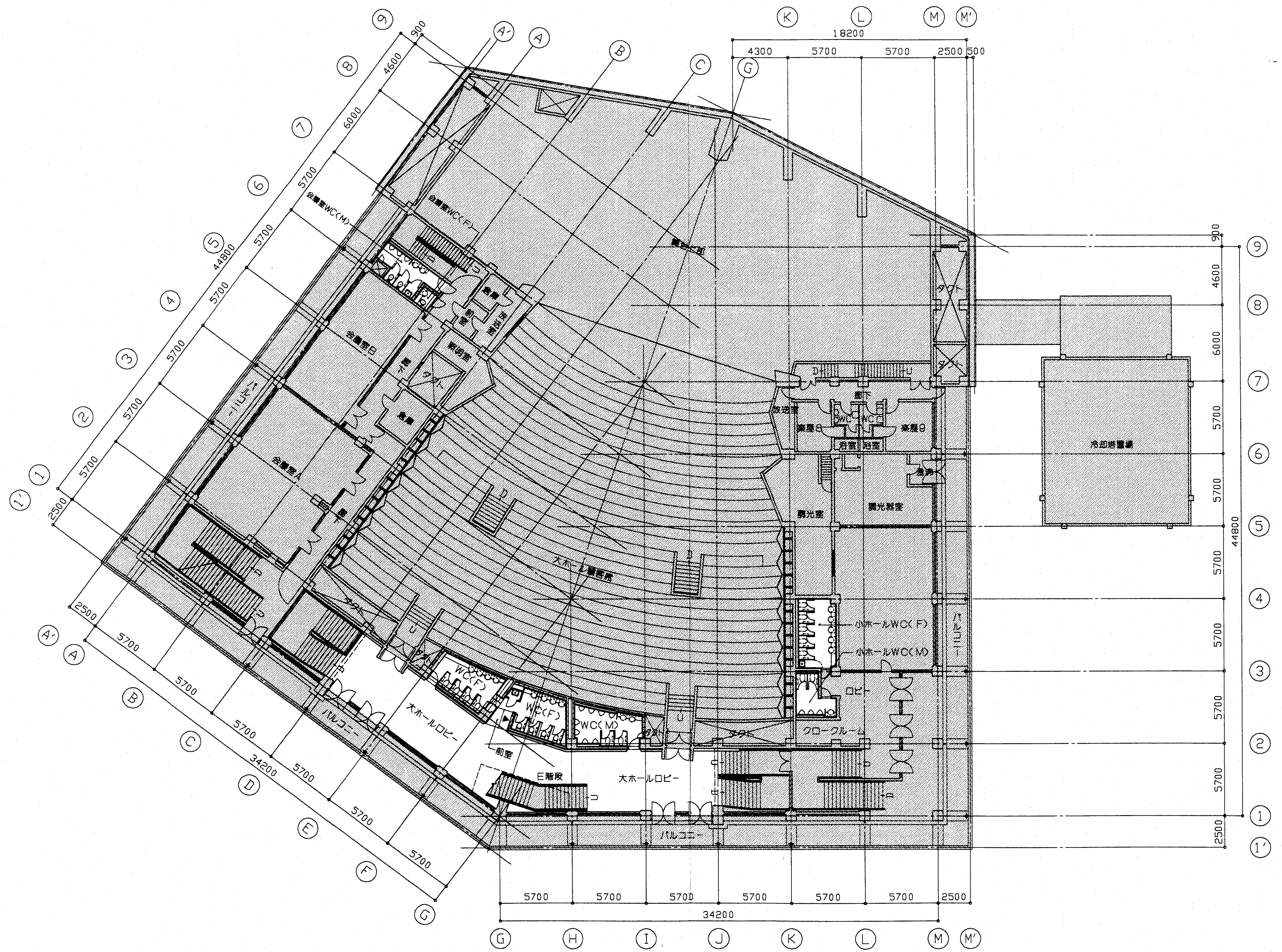
2階平面図
