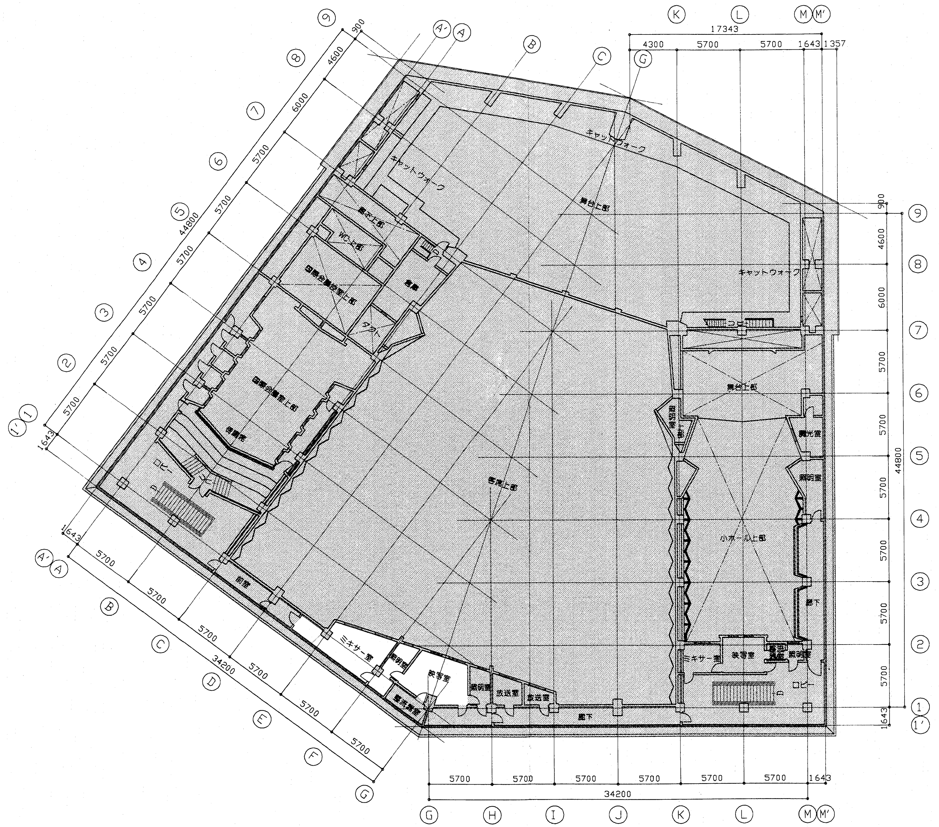
4階平面図
