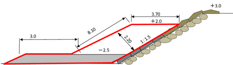
第2号突堤改良断面図(案)
