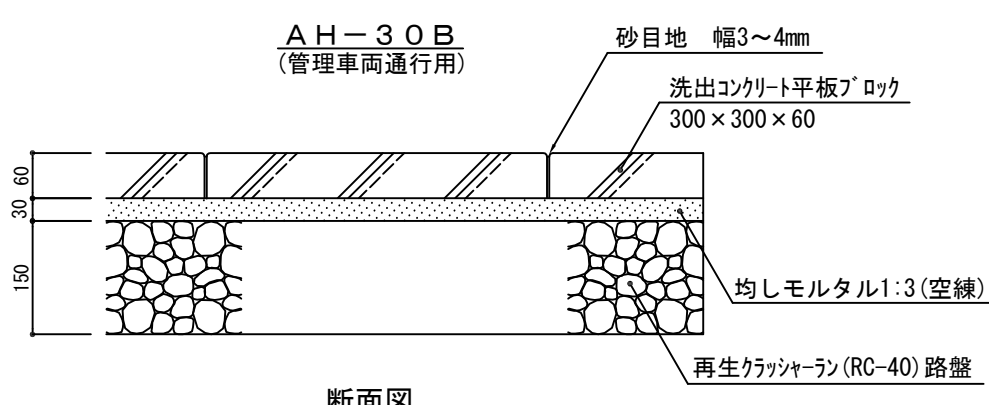
断面図
