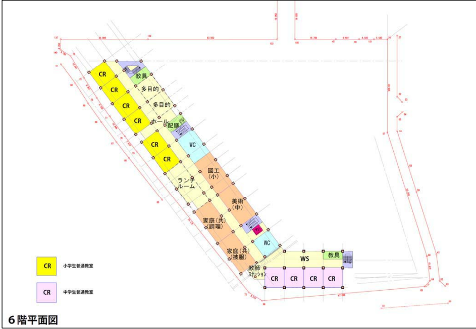
6階平面図
