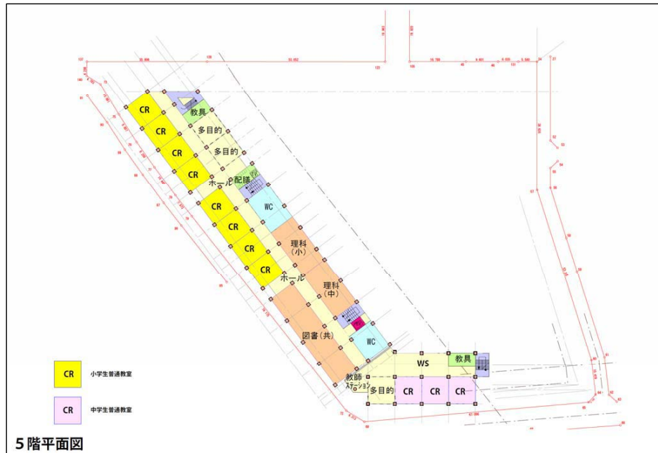
5階平面図
