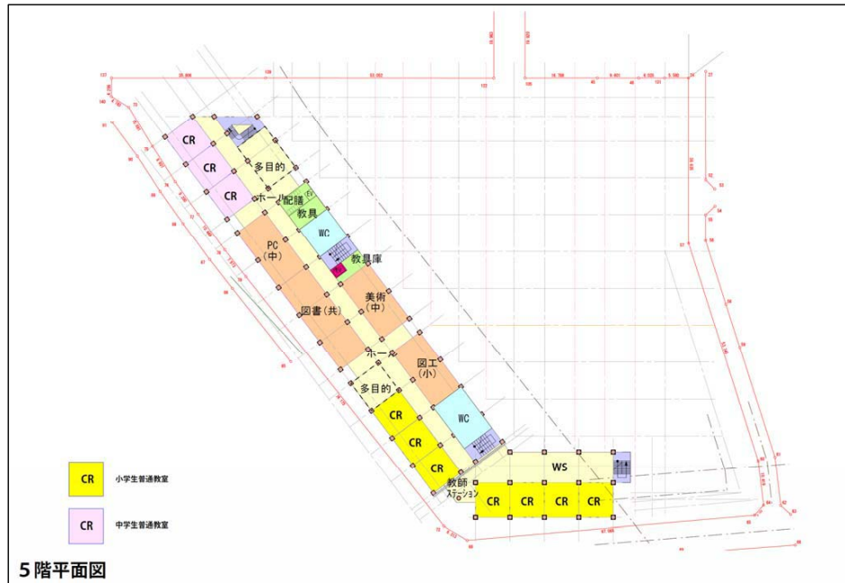
5階平面図
