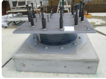
免震装置設置後の様子
